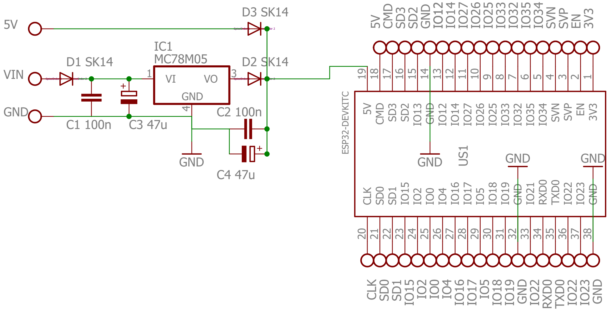
Easy Switch ES-7.01 NodeMCU ESP-32
